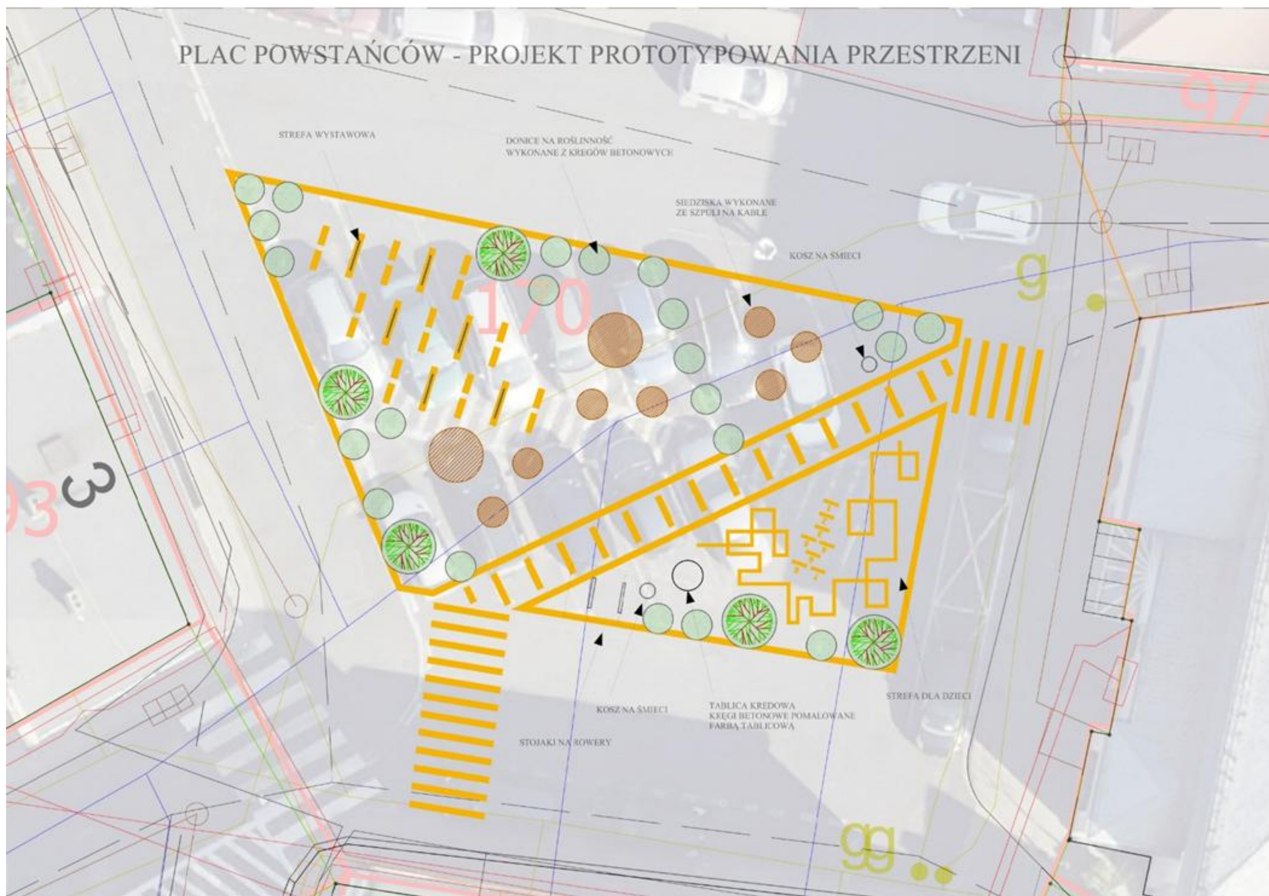
Rys.2 Projekt prototypowania placu (rzut z góry)
