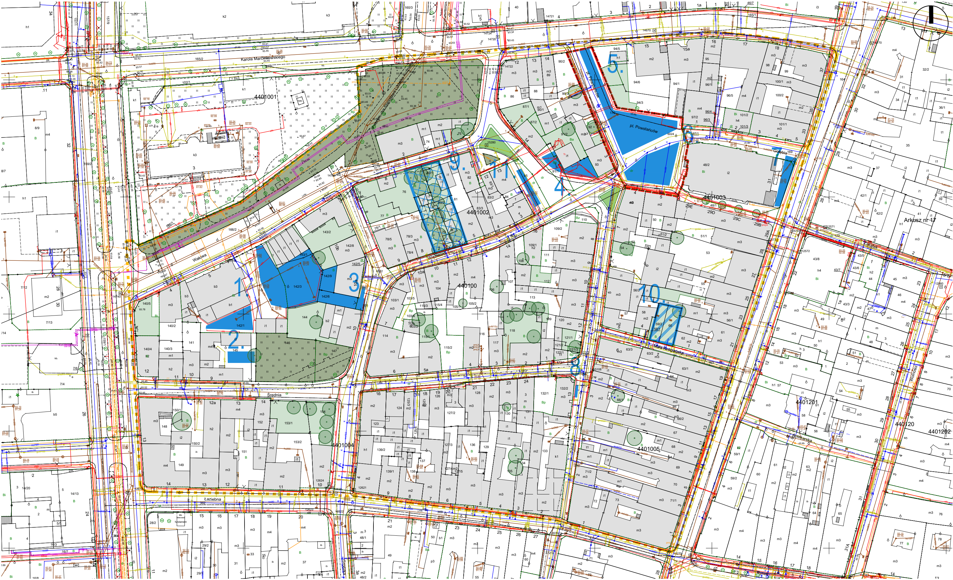
ANALIZA TERENÓW MOŻLIWYCH DO ODBETONOWANIA W KONTEKŚCIE INFRASTRUKTURY PODZIEMNEJ 1:1000
